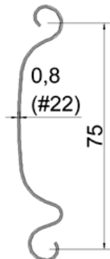
LÂMINAS DE, AÇO 0,788 Kg/m
