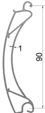
LÂMINA DUPLA (ALUMÍNIO) 0,784 Kg/m
