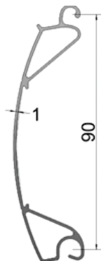
LÂMINA SIMPLES (ALUMÍNIO) 0,593 Kg/m
