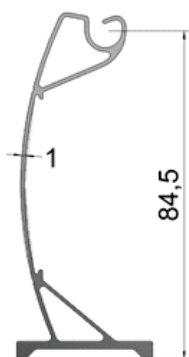
SOLEIRA (ALUMÍNIO) 0,723 Kg/m
